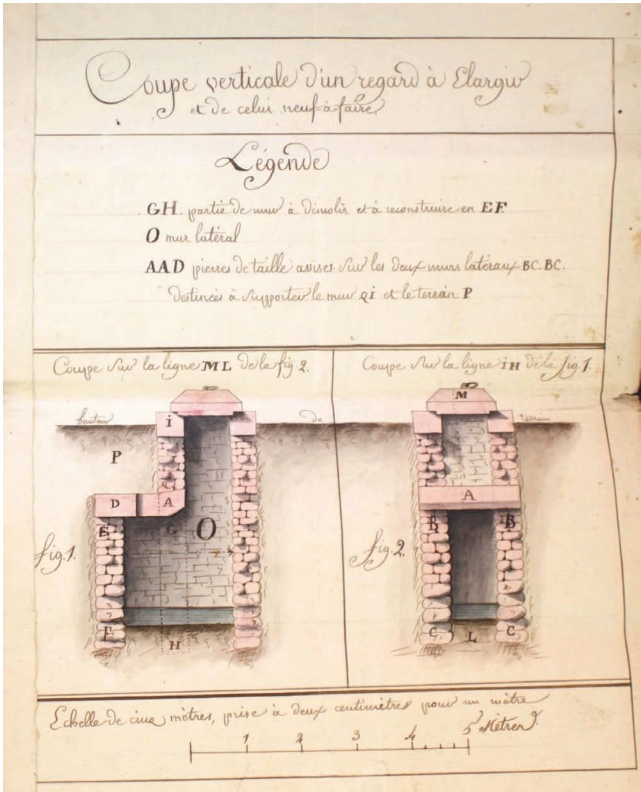
Coupe verticale de regards à élargir et à faire à la conduite de la fontaine du Théron (1819)
