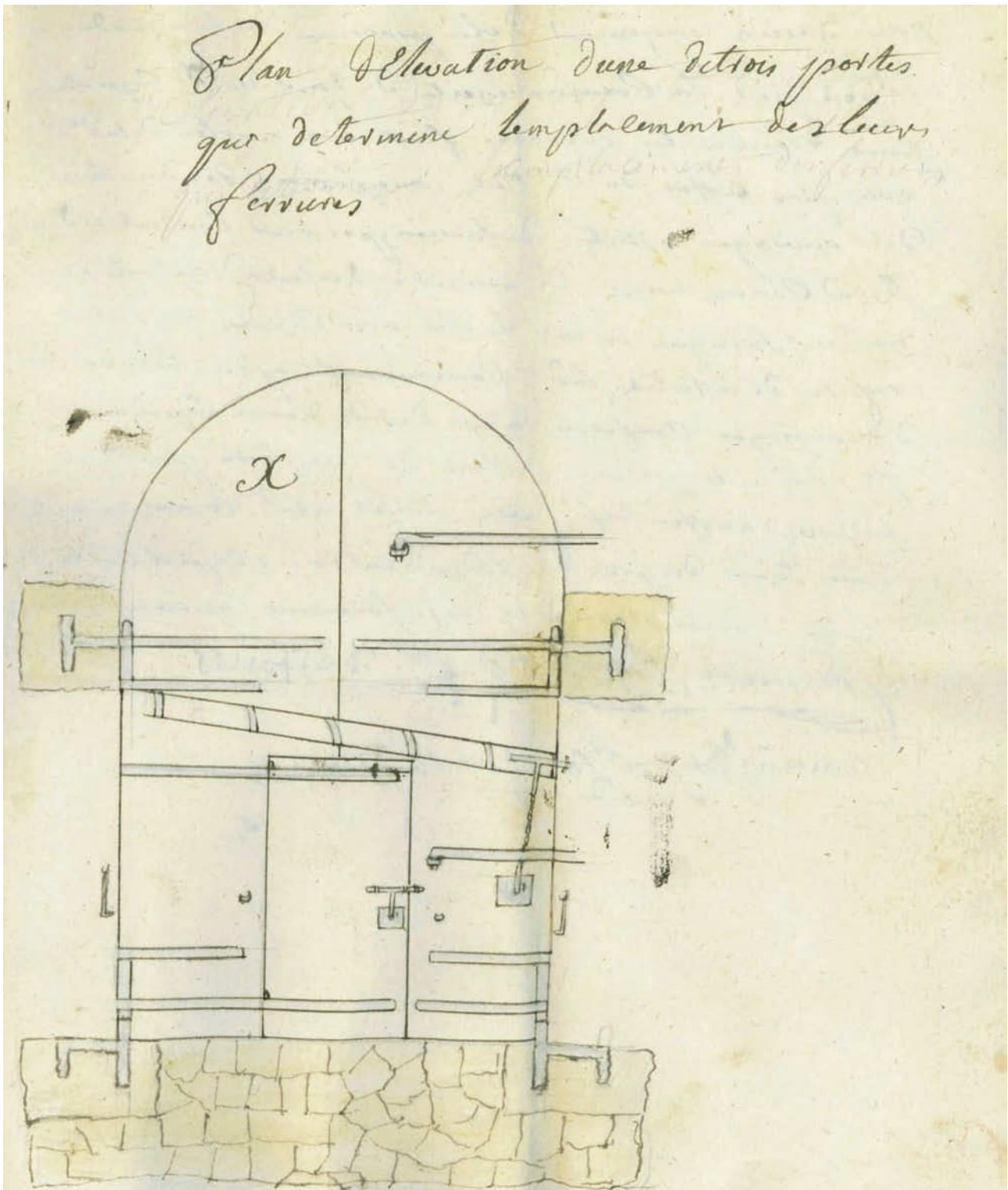
Plan d'élévation d'une des portes de la ville extrait d'un devis d'ouvrages de menuiserie et serrurerie à faire à trois portes de l'enceinte (1775) EE2
